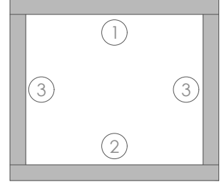
Glazing bead assembly sequence Cam çitası montaj sıralaması
